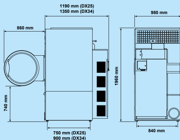
Seitenansicht DX 25 34
